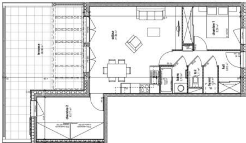
plan échelle 1/100
