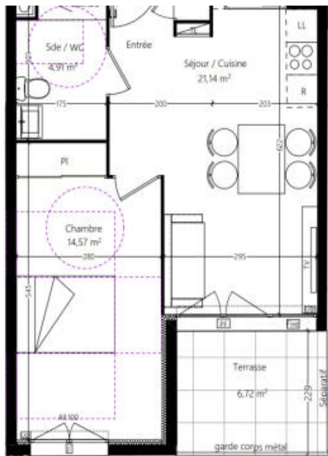
Plan Appartement
